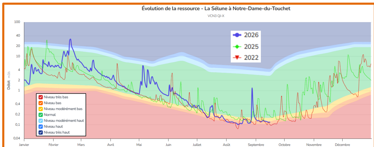
Figure 7 : Indicateur d'évolution des débits de la Sélune à Notre-Dame-du-Touchet au 16 septembre 2026
