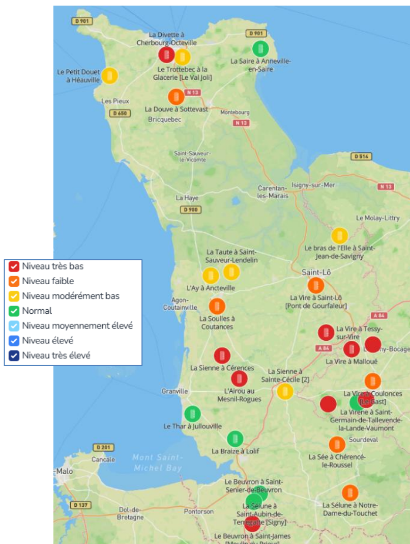
Figure 5 : Indicateur des débits des stations de jaugeage dans la Manche, situation au 16/09/2026
