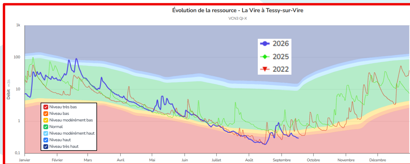
Figure 6 : Indicateur d'évolution des débits de La Vire à Tessy-sur-Vire au 16 septembre 2026
