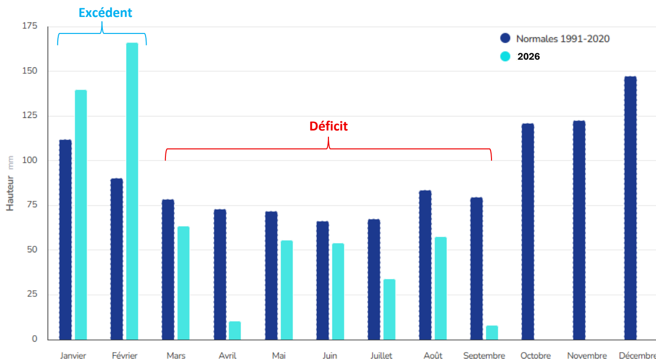
Figure 3 : Diagramme de cumul mensuel de précipitations en 2026 et comparaison aux normales (analyse réalisée sur la période 1991-2020) (METEO FRANCE – Cerisy-la-Salle) (Situation au 14/09/2026)
