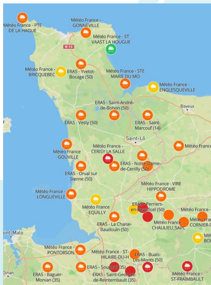
Figure 4 : Indicateurs de la température (°C) des 30 derniers jours. Situation au 01/09/2026 (Données actualisées du 29/08/2026)
