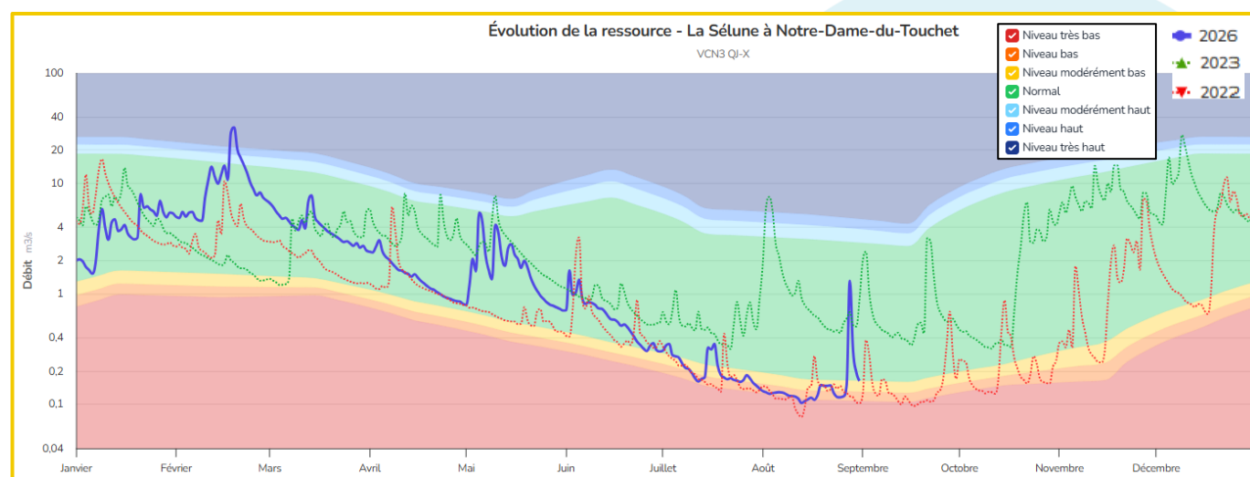
Figure 7 : Indicateur d'évolution des débits de la Sélune à Notre-Dame-du-Touchet au 01 septembre 2026
