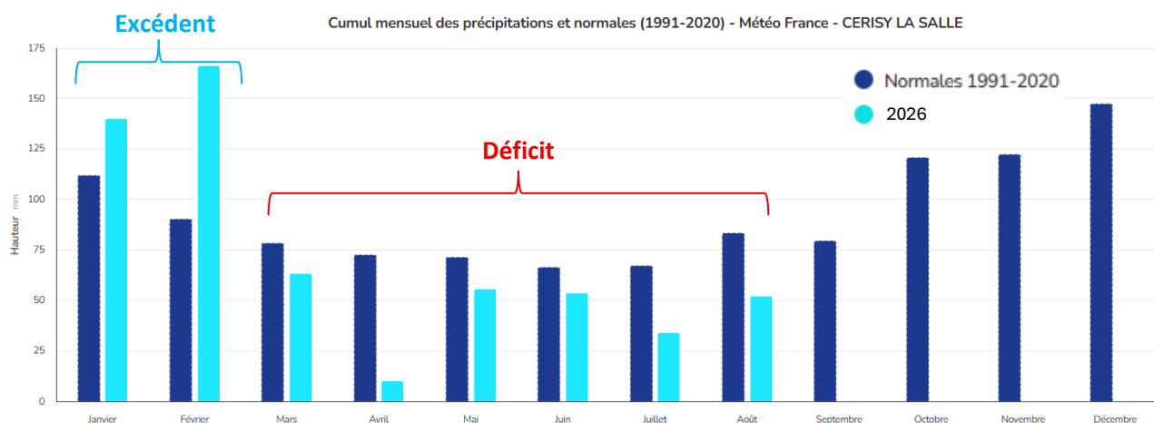
Figure 3 : Diagramme de cumul mensuel de précipitations en 2026 et comparaison aux normales (analyse réalisée sur la période 1991-2020) (METEO FRANCE – Cerisy-la-Salle) (Situation au 29/08/2026)
