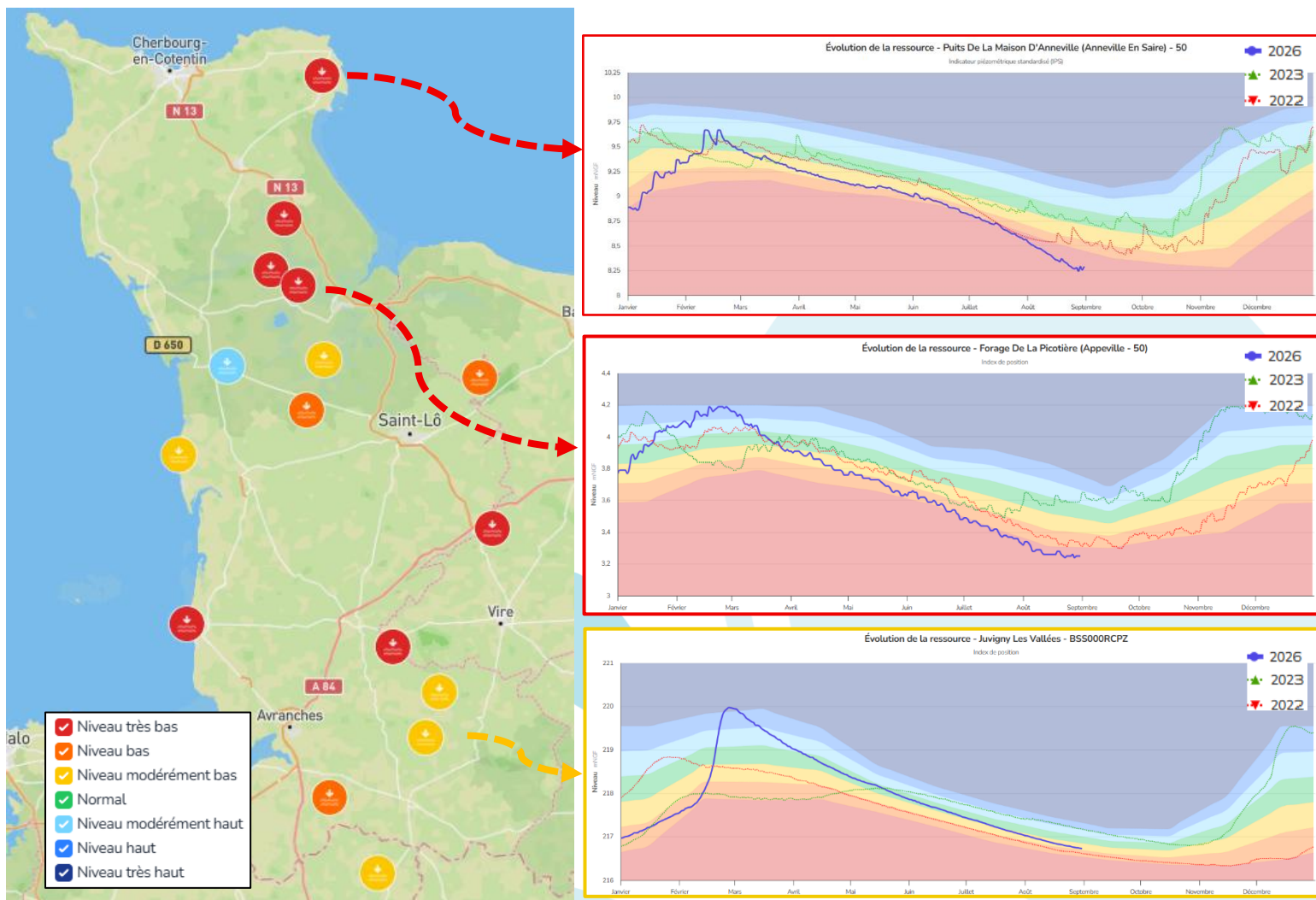
Figure 8 : Indicateur IPS des piézomètres dans la Manche (à gauche) et courbes de niveaux pour 3 piézomètres à Anneville-en-Saire, Appeville et Juvigny-les-Vallées (à droite). Situation au 01/09/2026 (Données actualisées du 31/08/2026).
