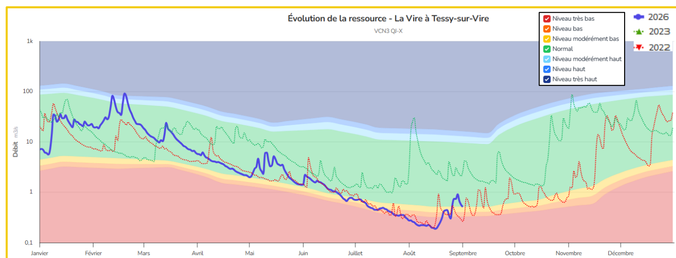
Figure 6 : Indicateur d'évolution des débits de La Vire à Tessy-sur-Vire au 01 septembre 2026
